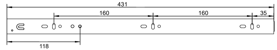
Innenschiene
