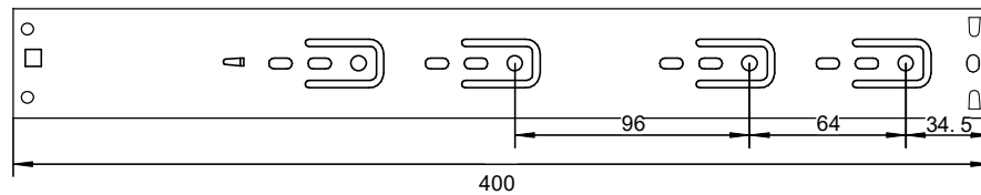
Außenschiene
