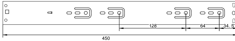
Außenschiene
