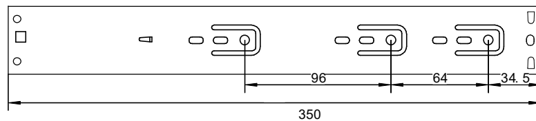
Außenschiene
