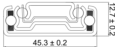
Seitenprofil
