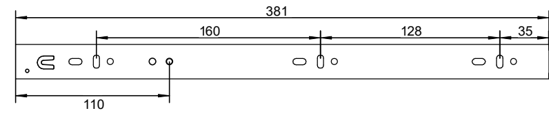
Innenschiene
